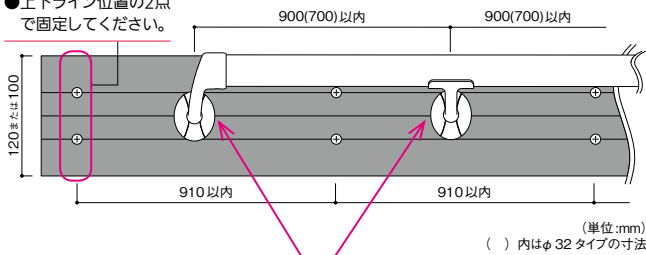
一般部 センターラインの位置にブラケットを固定してください。
