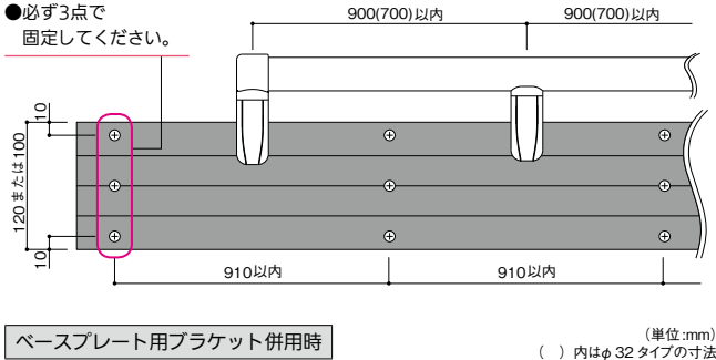
ベースプレート用ブラケット併用時
