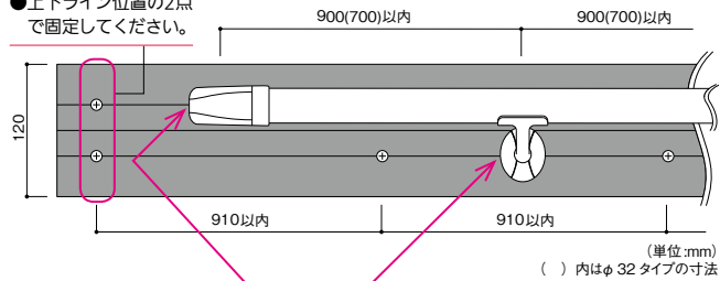
エンドブラケット併用時 上下ラインの位置にブラケットを固定してください。
